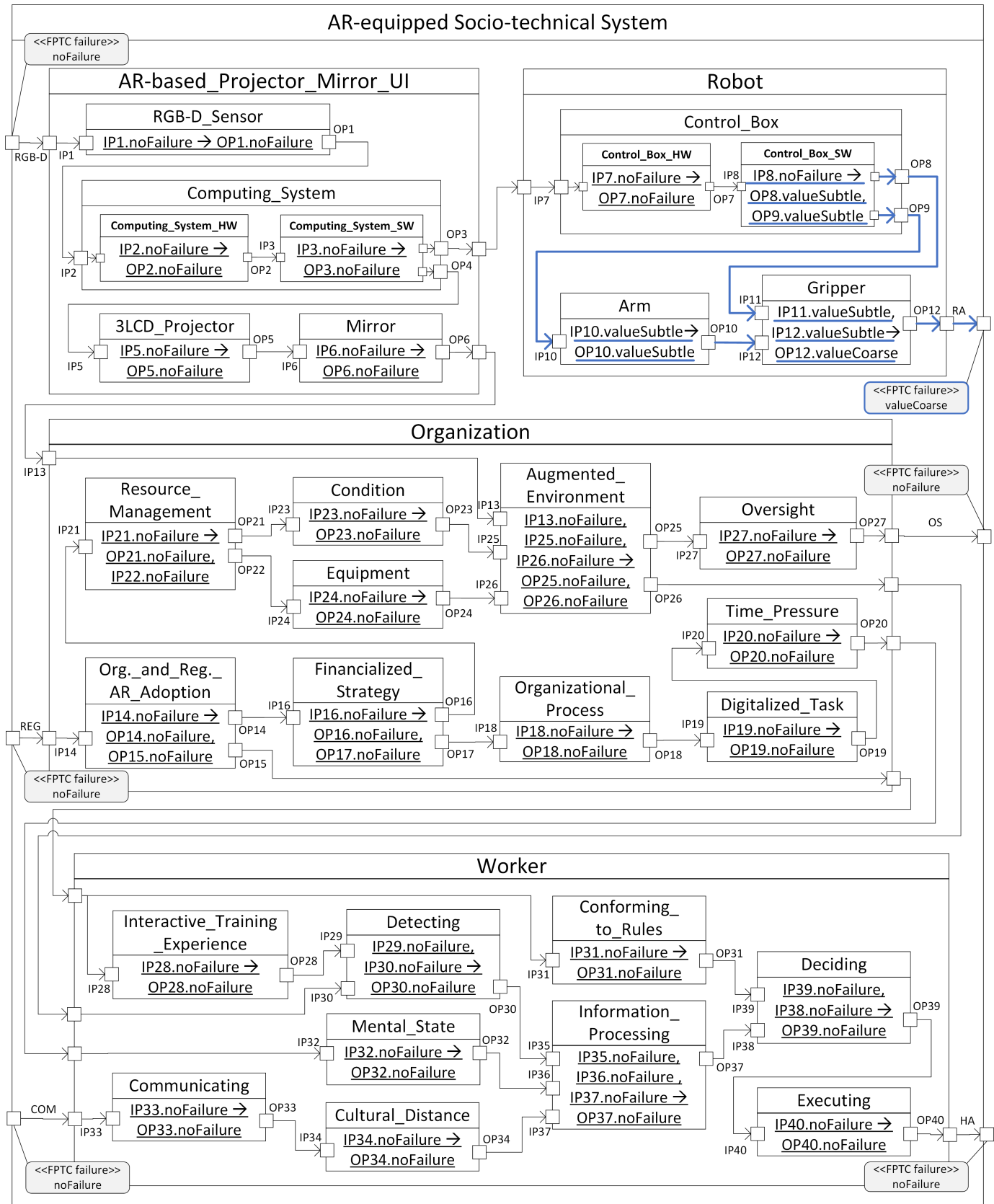
Fig. 13. Analyzing the AR-equipped socio-technical system (Scenario 3).
